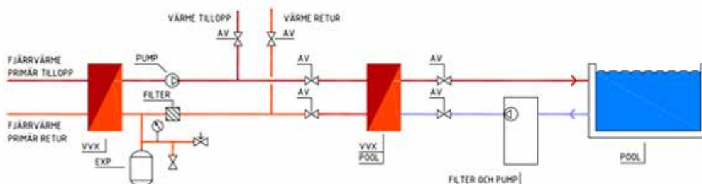
Figur 9. Sekundäransluten poolvärmesväxlare.
