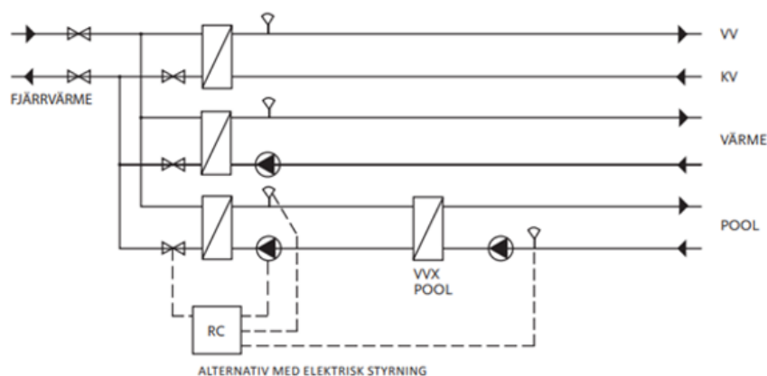
Figur 10. Separat primäransluten poolvärmewäxlare.
