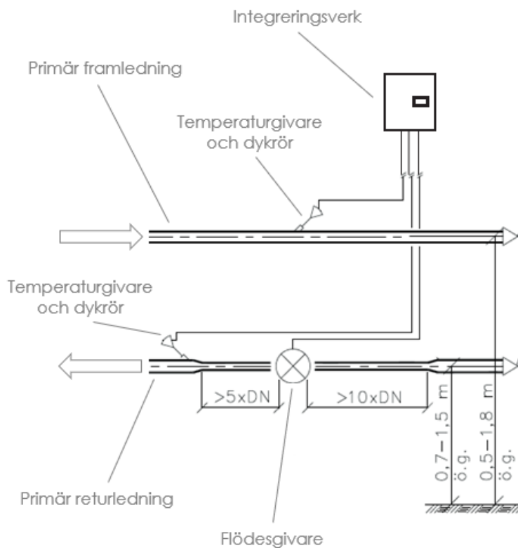
Figur 11. Princip över mätarplatsens utförande.
