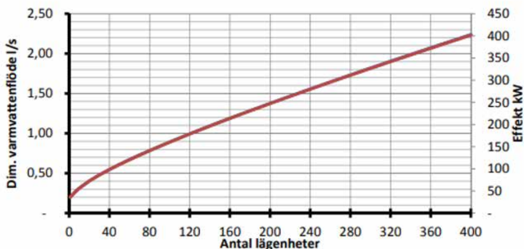
Figur 2. Dimensionerande varmvattenbehov vid nybyggnation.
