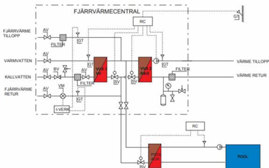
Figur 8. Primäransluten poolvärmesväxlare.
